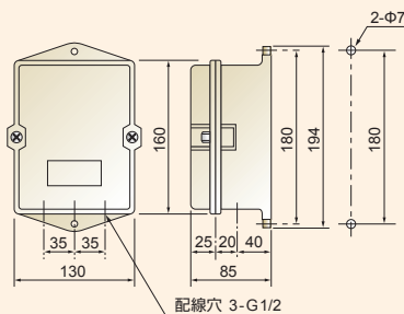
屋外用分離函
