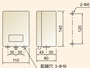
屋内用分離函
