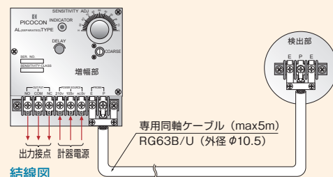
結線図
